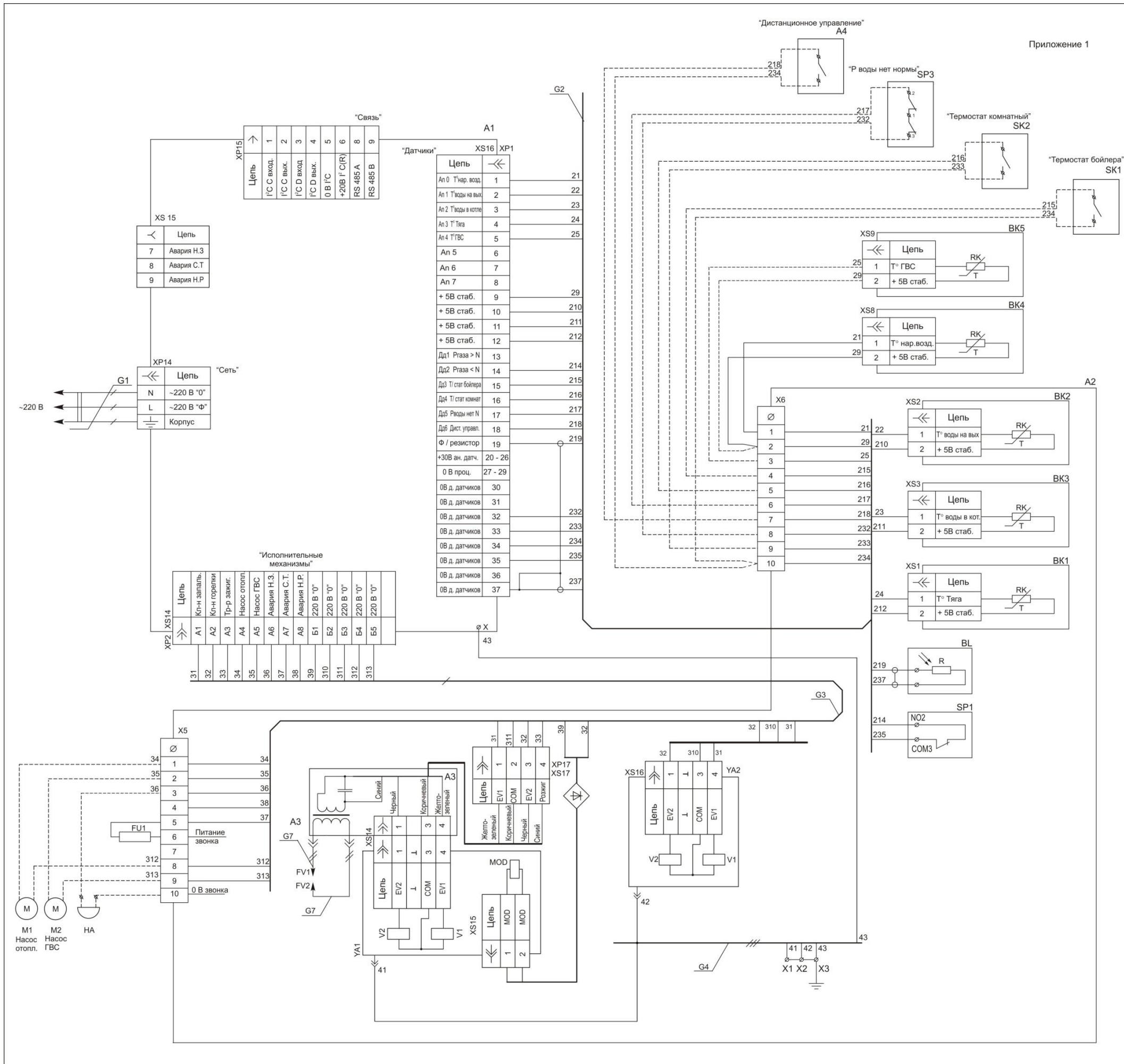
Котел водогрейный стальной модели "Хопер-А" Схема подключений
