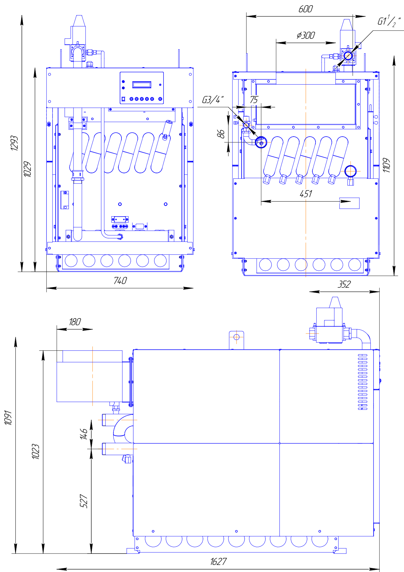
Рис. 1 Габаритные и присоединительные размеры
