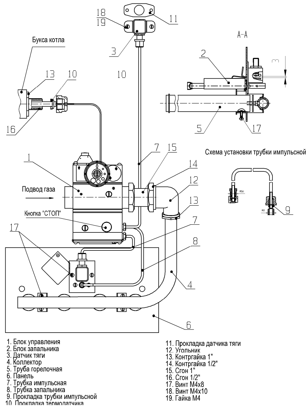
Рисунок 2 Монтаж автоматики САБК-М на котел
